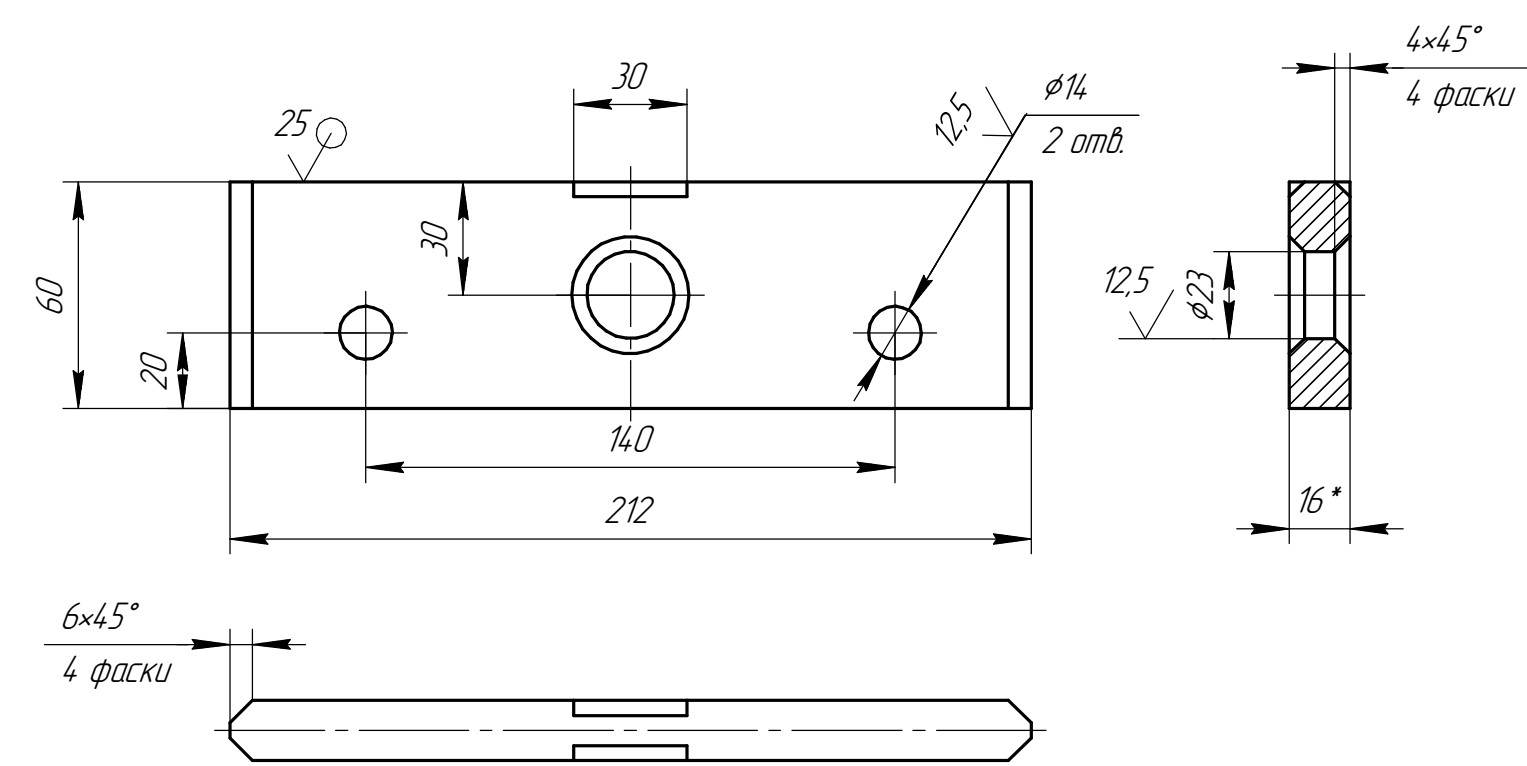
Дет. поз.11 (1:2)
