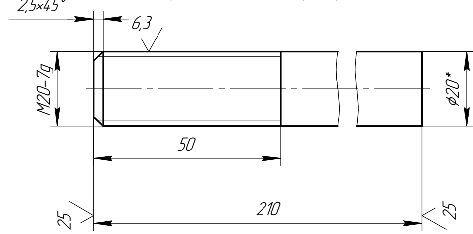
Дет. поз.5 (1:1)
