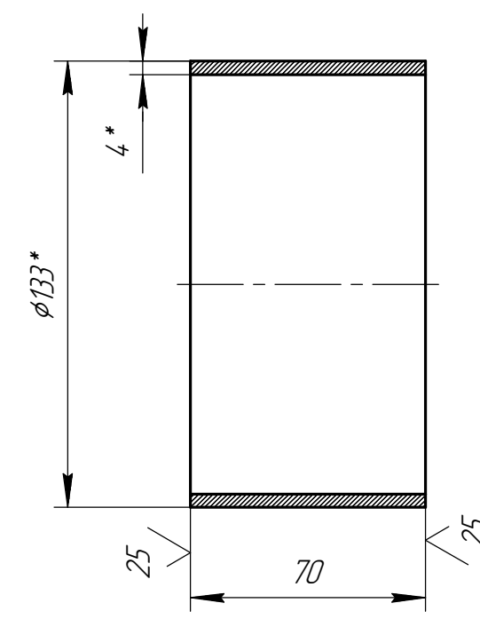
Дет. поз.9 (1:2)
