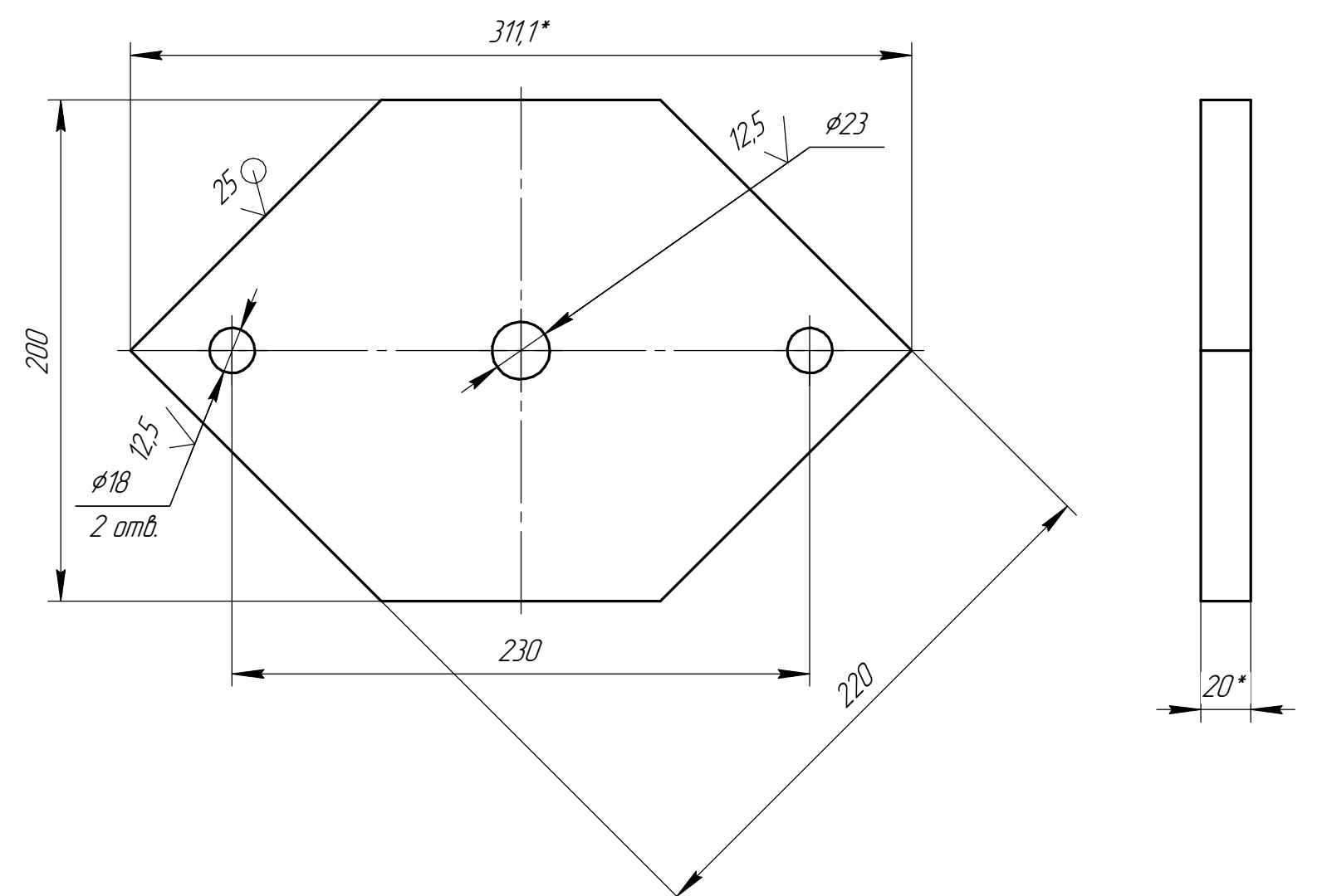
Дет. поз.9 (1:2)
