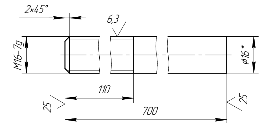
Дет. поз.10 (1:1)
