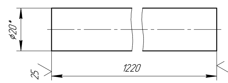
Дет. поз.12 (1:1)
