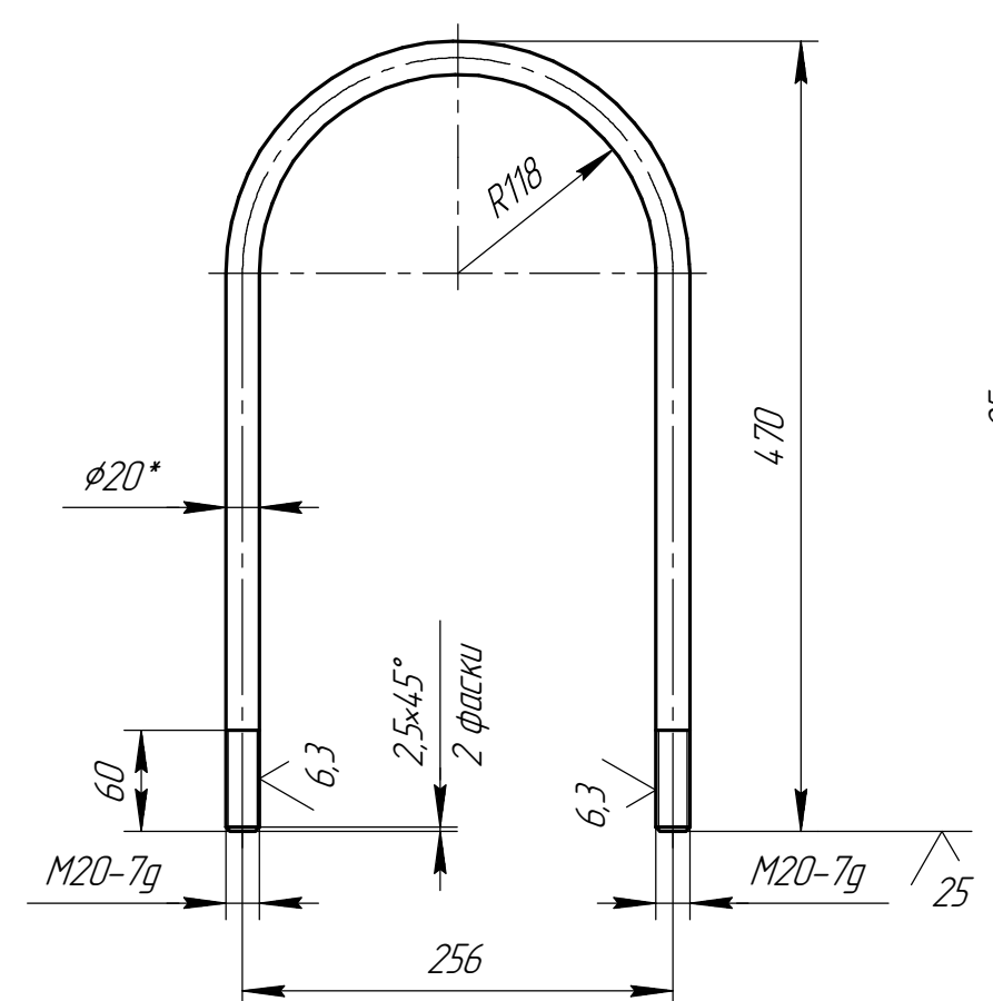
Дет. поз.1 (1:5)
