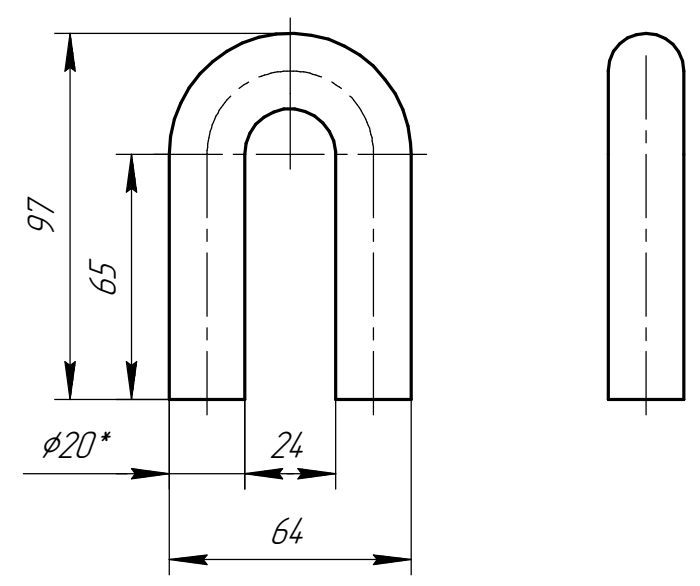
Дет. поз.6 (1:2)
