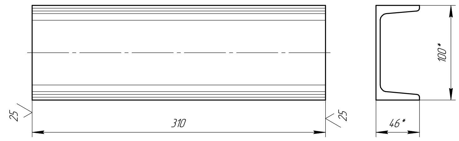
Дет. поз.5 (1:1)
