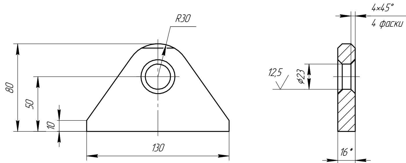
Дет. поз.13 (1:2)
