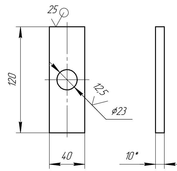
Дет. поз.3 (1:2,5)
