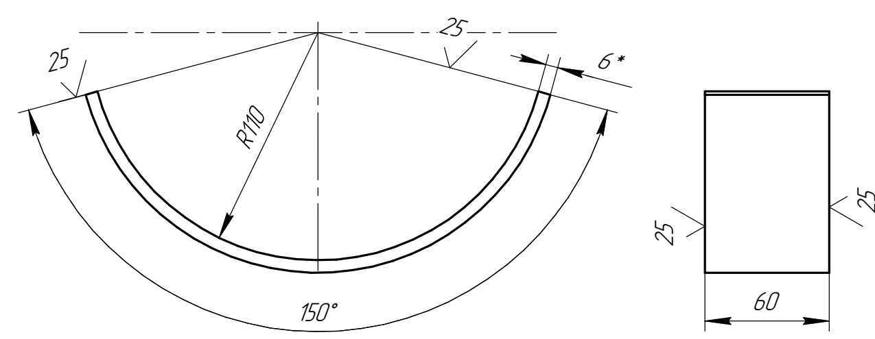
Дет. поз.2 (1:2,5)
