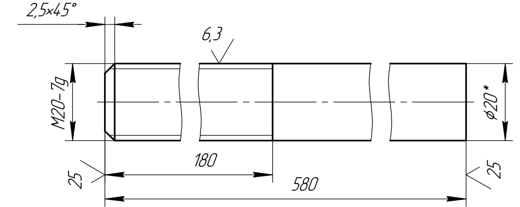
Дет. поз.7 (1:1)
